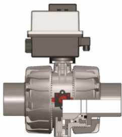
Шаровой кран VKD с эл.приводом 24V AC/DC, с удлиненными патрубками ПП (уплотнение EPDM) PP-H d90 (DN80)
