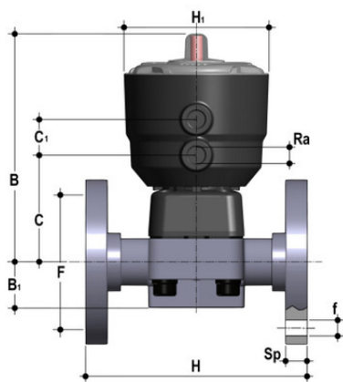
Мембранный клапан DK с пневмоприводом ДвД, PN10 с фланцевыми окончаниями (уплотнение FKM/мембрана PTFE) PP-H d20 (DN15)
