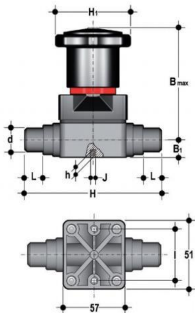
Компактный мембранный клапан СМ ПВХ с пневмоприводом НЗ, втулочные окончания, FKM, FIP d20 (DN15)
