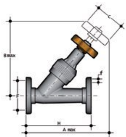
Угловой вентиль VVOV PBX с фланцевыми окончаниями, EPDM, FIP d50 (DN40)
