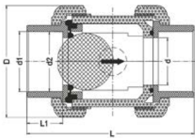
Обратный клапан шаровой с муфтовыми окончаниями PP-H IPS d40
