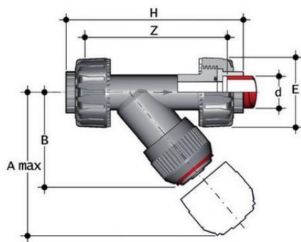
Грязевой фильтр RVUIM с муфтовыми окончаниями (уплотнение EPDM) PP-H d50 (DN40)
