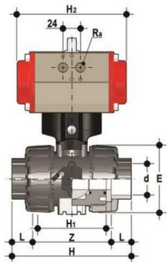
Шаровой кран VKD ПВХ с пневмоприводом НЗ с муфтовыми окончаниями, FKM, FIP d63 (DN50)
