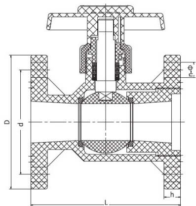
Шаровой кран IVKD ПВДФ с фланцевыми окончаниями d75 (DN65)
