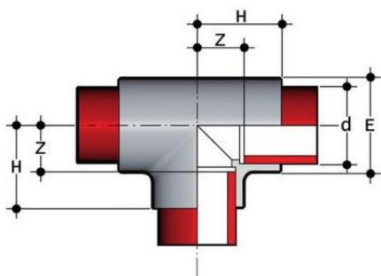
Тройник равнопроходной для раструбной сварки PP-H FIP d32 PN10
