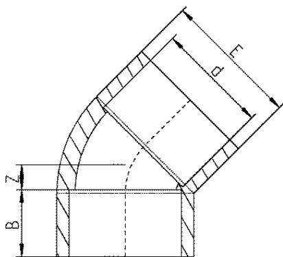
Отвод клеевой 45° ПВХ Praher Plastics d12
