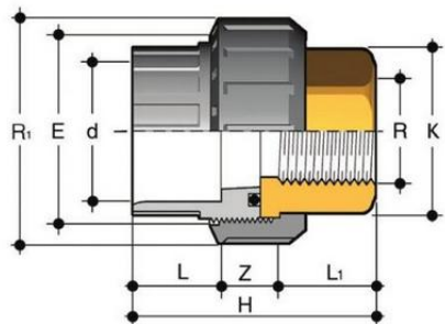
Муфта разборная ХПВХ/ латунь, ВР 32х1" PN16
