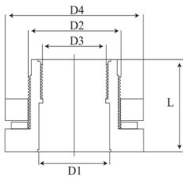
Соединитель с цистерной, ILIFV ПВХ IPS d75
