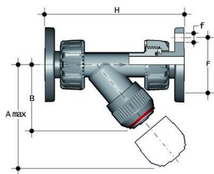
Грязевой фильтр RV ХПВХ с фланцевыми окончаниями d20 (DN15)
