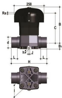
Мембранный клапан VM ХПВХ с пневмоприводом НЗ с втулочными окончаниями d110 (DN90)
