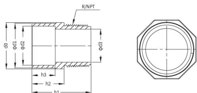
Редукционная муфта ПВДФ с НР для стыковой сварки 63х2" PN 16
