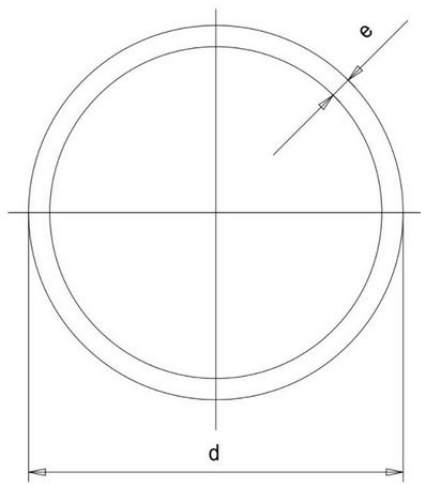
Напорная труба РР-Н Симона, PN6 d315
