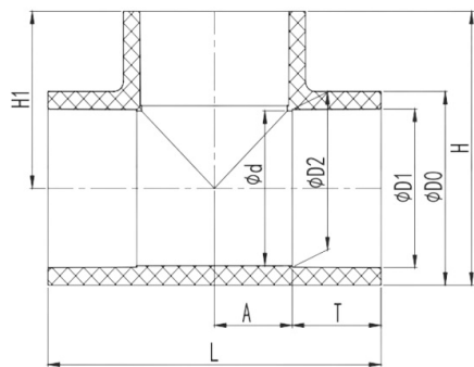
Тройник равнопроходной клеевой 90° ПВХ IPS d25
