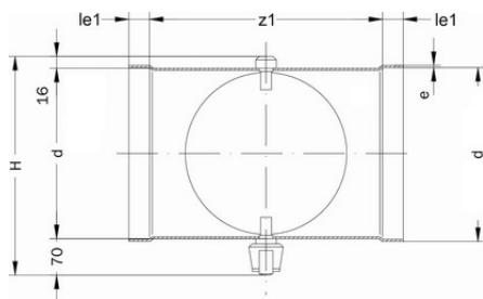
Дроссельный клапан с плавной регулировкой PPs d225
