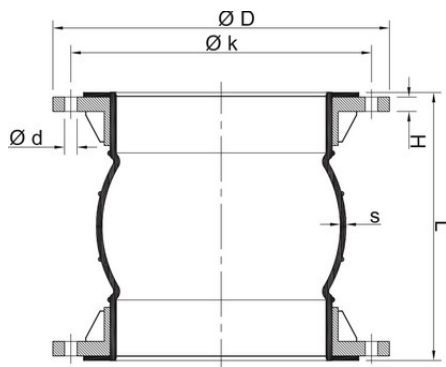
Шаровая манжета с фланцами PPs d160
