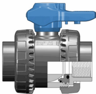
Шаровой кран ПВХ общего применения VEE; муфтовые окончания с ВР, EPDM, FIP R1/2" (DN15)
