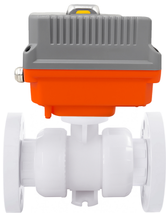
Шаровой кран IVKD ПВДФ с эл.приводом 220V AC, фланцевые окончания, EPDM, IPS d25 (DN20)
