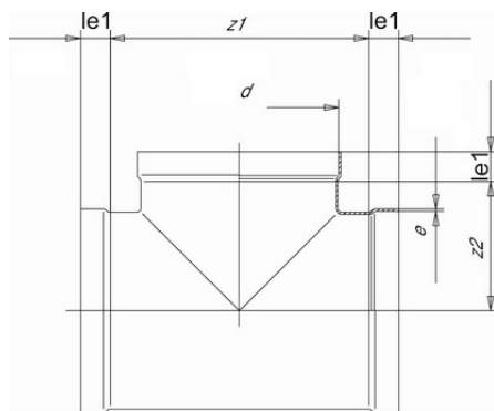
Тройник равнопроходной PPs d50
