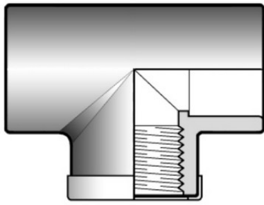
Тройник переходной с НР ПВХ FIP 40x1 1/4
