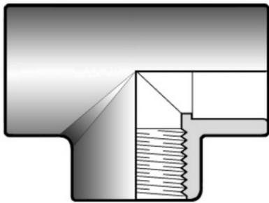
Тройник переходной с ВР ПВХ FIP 63x1/2
