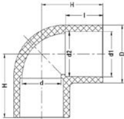
Отвод 90° ХПВХ IPS (Model A) d32 PN16
