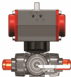
3-х ходовой шаровой кран ТКД с пневмоприводом ДвД с муфтовыми окончаниями, L-шар (уплотнение EPDM) PP-H d40 (DN32)
