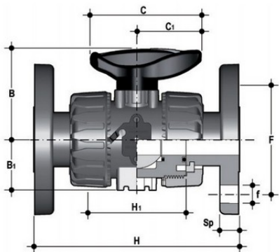
Шаровой кран ПВХ промышленного применения VKD с фланцевыми окочаниями, FKM, FIP d75 (DN65)
