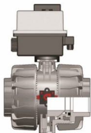
Шаровой кран VKD ПВХ с эл.приводом 90-240V, муфтовые окончания, DN65-100, FKM, FIP d90 (DN80)
