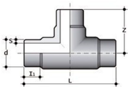
Тройник равнопроходной для стыковой сварки PP-H FIP d160 SDR17.6 PN10
