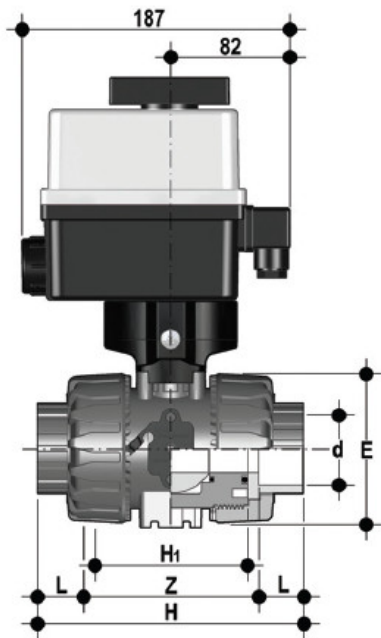
Шаровой кран VKD ПВХ с эл.приводом 24V AC/DC, муфтовые окончания, EPDM, FIP d50 (DN40)
