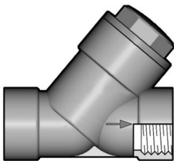
Угловой обратный клапан VRFV PBX с резьбовыми окончаниями, EPDM, FIP R2½" (DN65)
