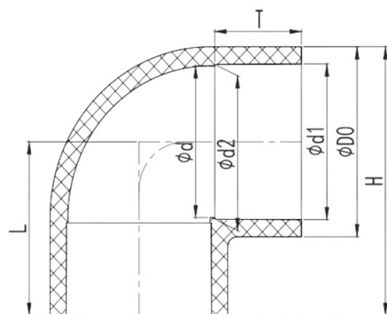
Отвод клеевой 90° ПВХ IPS d280
