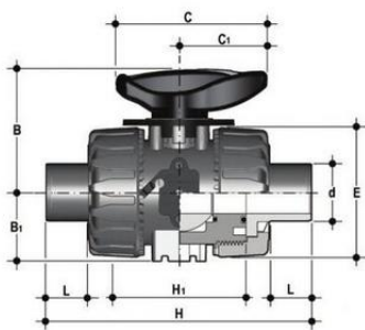
Шаровой кран для регулирования потока VKRDM с муфтовыми окончаниями (уплотнение FKM) PP-H d25 (DN20)
