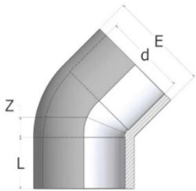
Отвод 45° ХПВХ Comer d110 PN16
