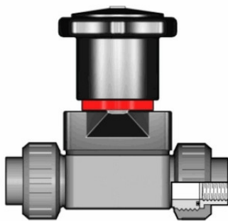
Компактный мембранный клапан CM ПВХ с пневмоприводом ДвД, резьбовые окончания, EPDM, FIP R1/2" (DN15)
