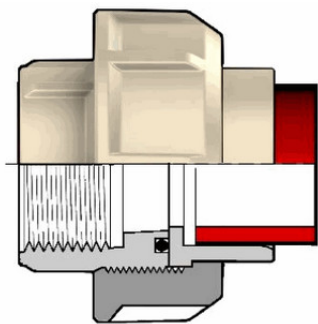
Разборная муфта с ВР, раструбная сварка РР-Н (EPDM) FIP 32x1 PN10
