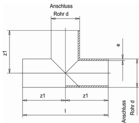
Тройник ПВХФ 90° (Simona) d32 SDR21 PN16
