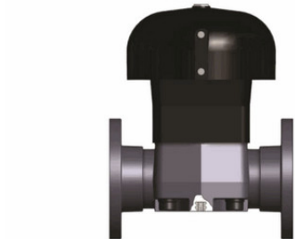
Мембранный клапан VM с пневмоприводом ДвД, PN10 с фланцевыми окончаниями (уплотнение FKM/мембрана PTFE) PP-H d90 (DN80)
