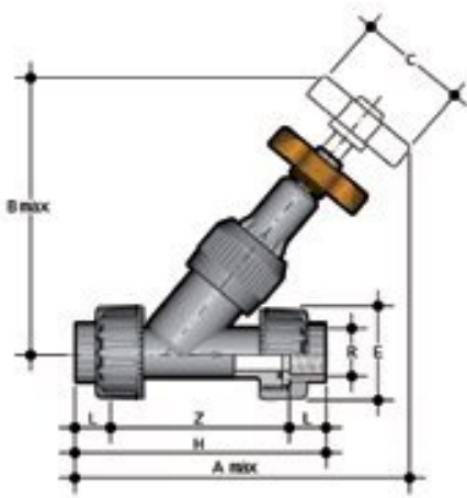
Угловой вентиль VUFV ПВХ с резьбовыми окончаниями, EPDM, FIP R1¼" (DN32)
