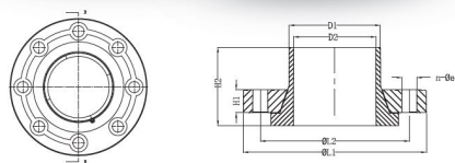
Бурт ПВДФ для стыковой сварки d225 PN 16
