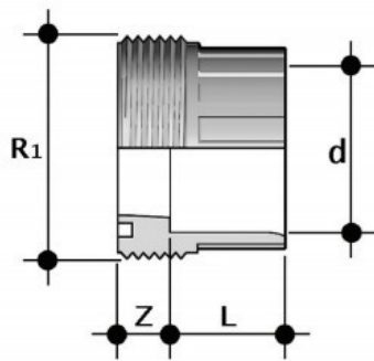
Муфтовая вставка для ВIV ПВХ FIP d63
