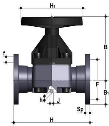
Мембранный клапан VMOM с фланцевыми окончаниями (уплотнение PTFE / мембрана PTFE) PP-H d90 (DN80)
