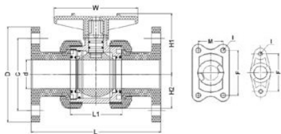
Кран шаровый ХПВХ фланцевые окончания промышленный FKM IPS d63 (DN50)
