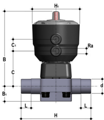
Мембранный клапан DK с пневмоприводом НО, PN10 с втулочными окончаниями (уплотнение FKM/мембрана FKM) PP-H d25 (DN20)
