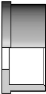
Муфтовое окончание для ВIV ПВХ FIP d10
