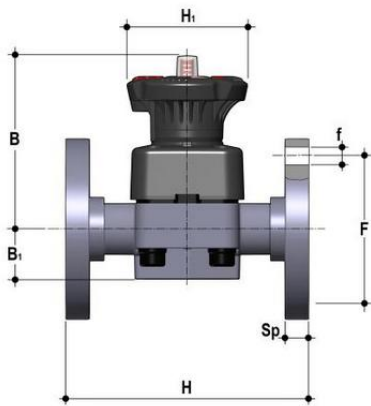
Мембранный клапан DKOV ПВХ с фланцевыми окончаниями, PTFE, FIP d25 (DN20)
