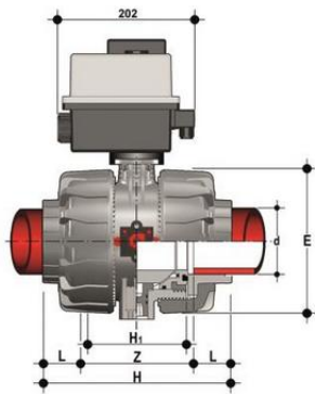
Шаровой кран VKD с эл.приводом 90-240V, муфтовые окончания, DN65-100 (уплотнение EPDM) PP-H d90 (DN80)
