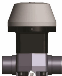
Мембранный клапан VM с пневмоприводом НЗ с втулочными окончаниями (уплотнение EPDM/мембрана EPDM) PP-H d90 (DN80)
