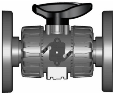
Шаровой кран ПВХ промышленного применения VKD с фланцевыми окочаниями, EPDM, FIP d50 (DN40)
