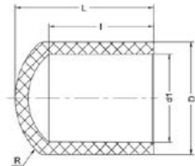
Заглушка для стыковой сварки PP-H IPS d25 PN10
